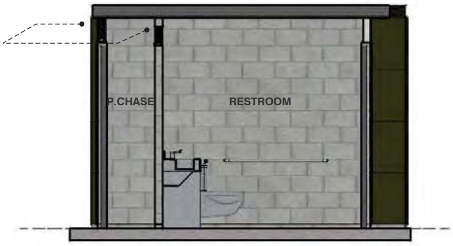
LONGITUDINAL SECTION
