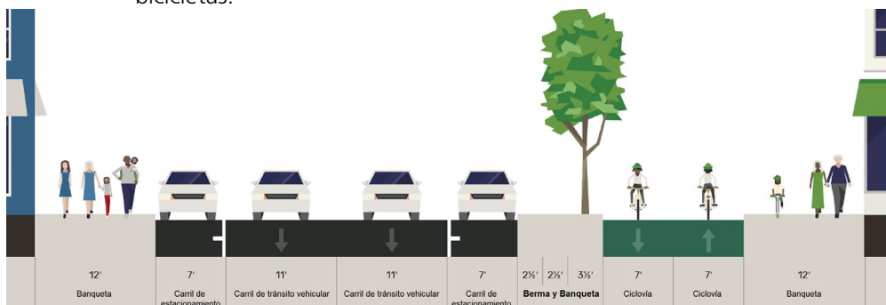
Típica sección transversal del proyecto Howard Streetscape
