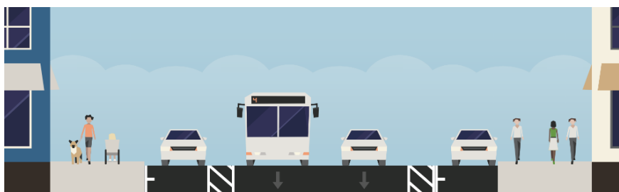
УЛИЦА LEAVENWORTH В РАЗРЕЗЕ: ПРЕДЛОЖЕННЫЕ
