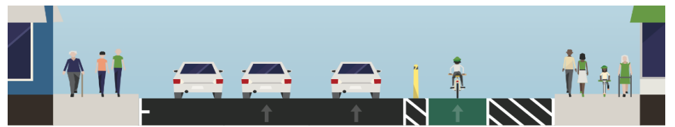
УЛИЦА GOLDEN GATE В РАЗРЕЗЕ: ПРЕДЛОЖЕННЫЕ
