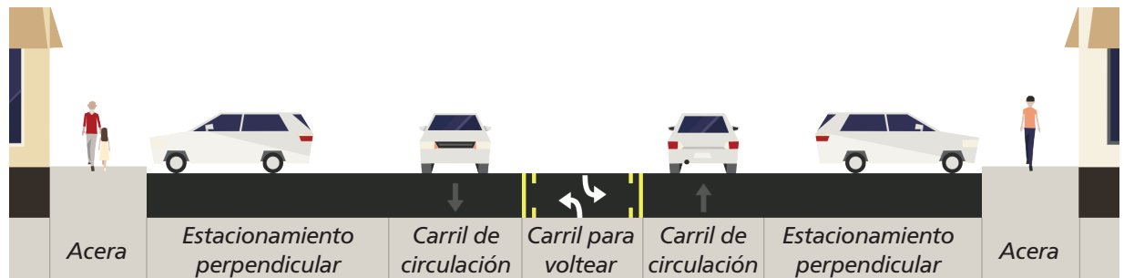
Configuración típica propuesta de la calle (mirando hacia el oeste)
