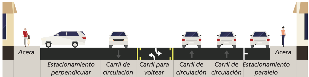
Configuración típica existente de la calle (mirando hacia el oeste)
