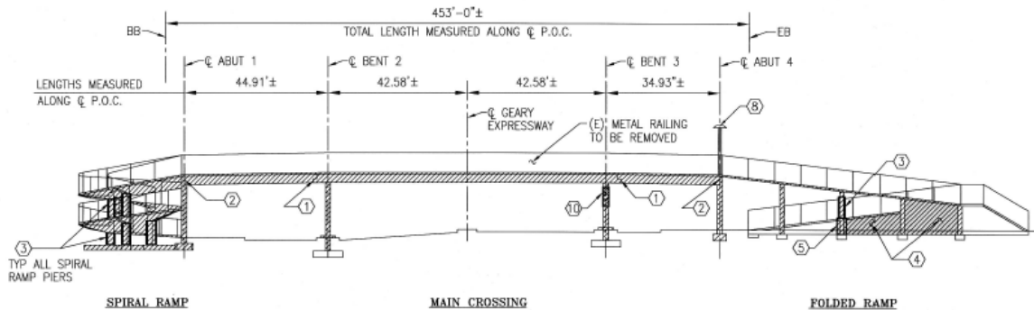
ELEVATION SCALE: 1"=20'
