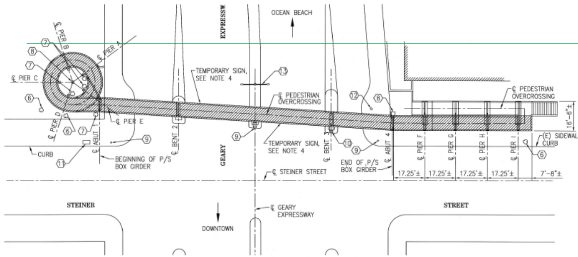
PLAN SCALE: 1"=20'
